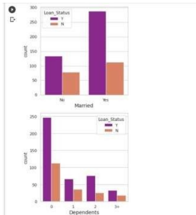
Fig.9. Missing Values
